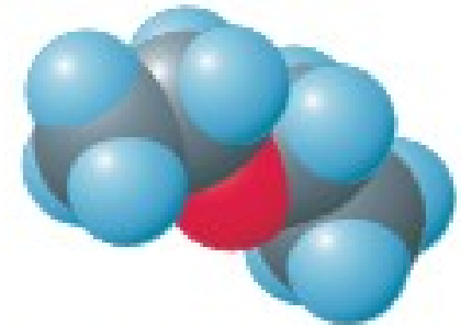
\text{CH}_3\text{CH}_2\text{OCH}_2\text{CH}_3 Diethyl ether
